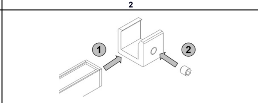
FISSAGGIO CON STAFFA MAGNETICA MAGNETIC BRACKET
