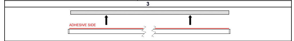
FISSAGGIO MAGNETICO - Magnets fixing
