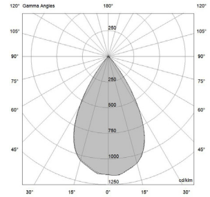
35W - 60° | UGR 22
