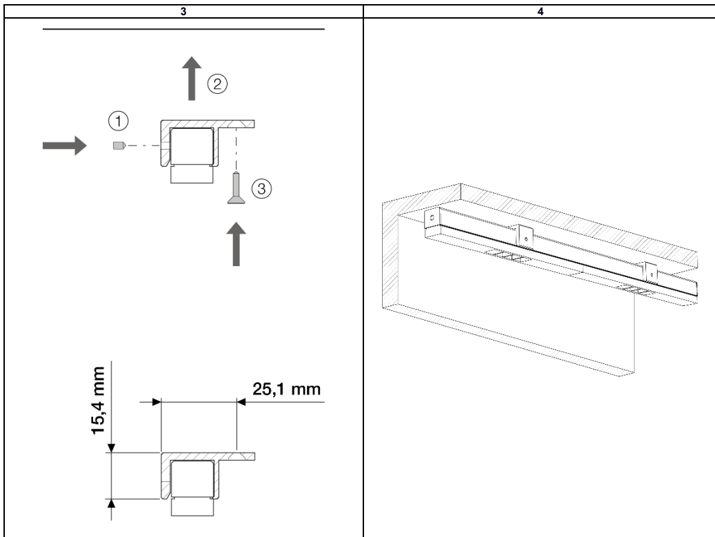
FISSAGGIO CON STAFFA MAGNETICA MAGNETIC BRACKET
