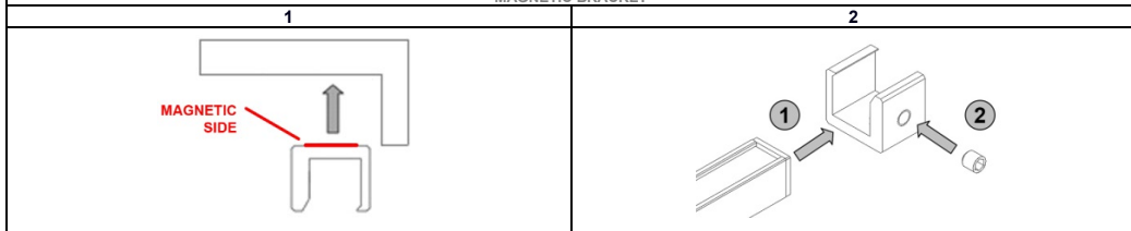
FISSAGGIO CON STAFFA MAGNETICA MAGNETIC BRACKET
