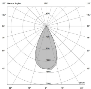
9W - 52° | UGR 19.4
