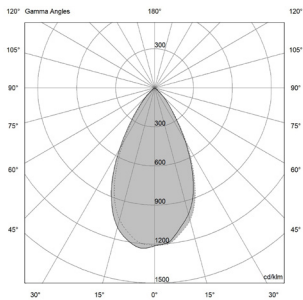
9W - 52° | UGR 22.2
