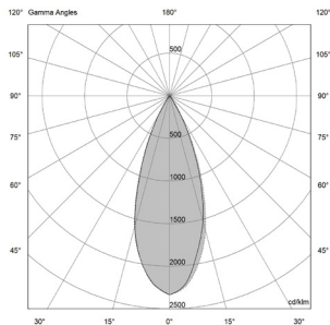
9W - 52° | UGR 13
