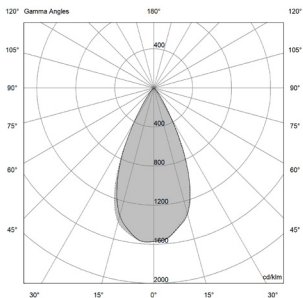
9W - 52° | UGR 18.9
