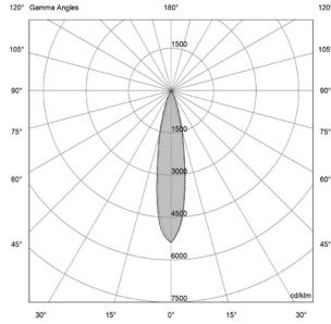
9W - 18° | UGR 9.6
