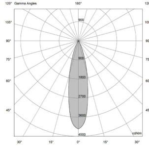
9W - 24° | UGR 11.8
