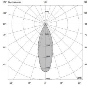
9W - 18° | UGR 15.6
