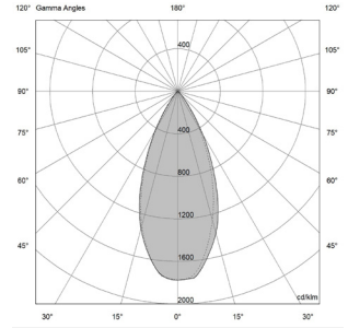
9W - 33° | UGR 17.8
