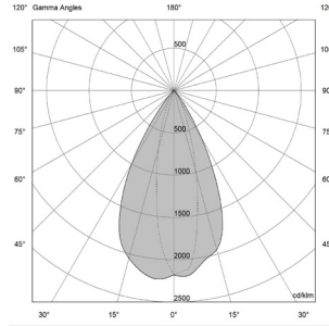
9W - 24° | UGR 8.9
