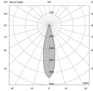
9W - 24° | UGR 8.7
