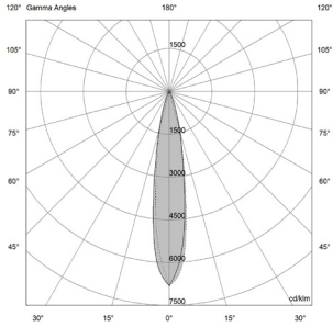
9W - 14° | UGR 7.8
