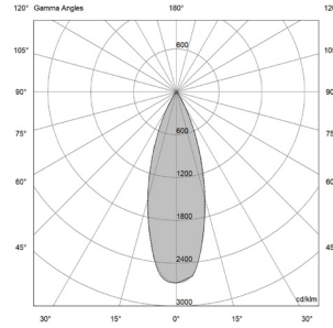
9W - 33° | UGR 14.1
