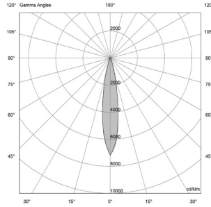
9W - 18° | UGR 4.2
