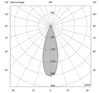
9W - 33° | UGR 12.4
