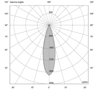
9W - 33° | UGR 8.4
