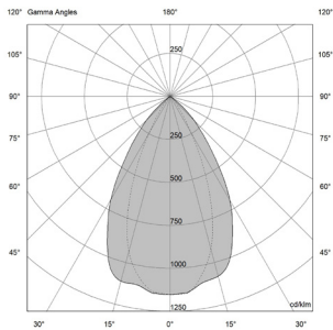
9W - 52° | UGR 18.3
