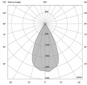
9W - 18° | UGR 9.5
