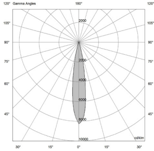
9W - 14° | UGR 6.1
