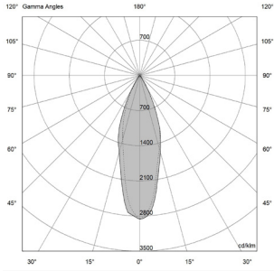
9W - 14° | UGR 13.8
