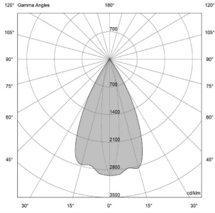
9W - 14° | UGR 8.5
