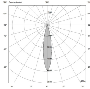
9W - 24° | UGR 6
