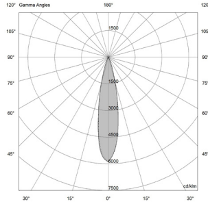
9W - 18° | UGR 6.4
