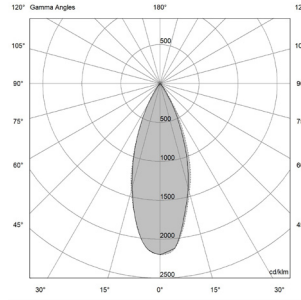
9W - 24° | UGR 16
