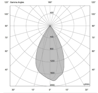
9W - 33° | UGR 13.6
