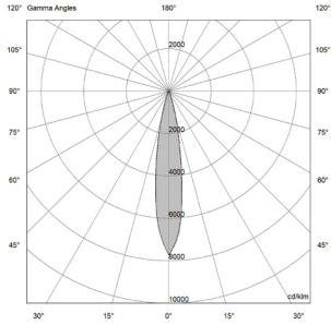
9W - 14° | UGR 4.1
